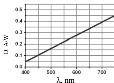
Rys. 7. Charakterystyka spektralna przykładowego, kalibrowanego fotodetektora typu FSD100-CAL produkcji Hamamatsu: \lambda – długość fali, D – czułość
