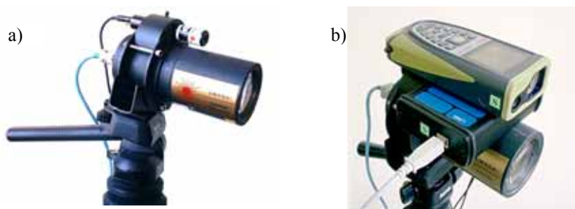
Fot. 2. Radiometr UV do zdalnego pomiaru pełnego strumienia promieniowania UV, w wersji z celownikiem laserowym (a) i dalmierzem (b); opracowany w GIG (2006 i 2008)
