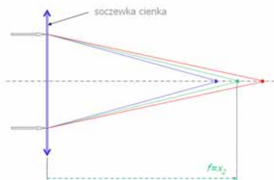
Rys. 2. Aberracja chromatyczna soczewki cienkiej
