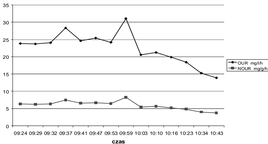
Rys. 2. Szybkość pobierania tlenu (OUR) oraz jednostkowa szybkość pobierania tlenu, przeliczona z uwzględnieniem stężenia osadu czynnego (NOUR) – pomiar prowadzony w fazie nityfikacji
