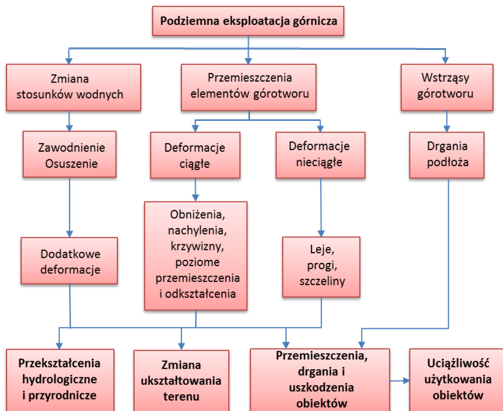
Rys. 1. Elementy kształtujące wpływ podziemnej eksploatacji górniczej na powierzchnię (Kwiatk red. 1998)
