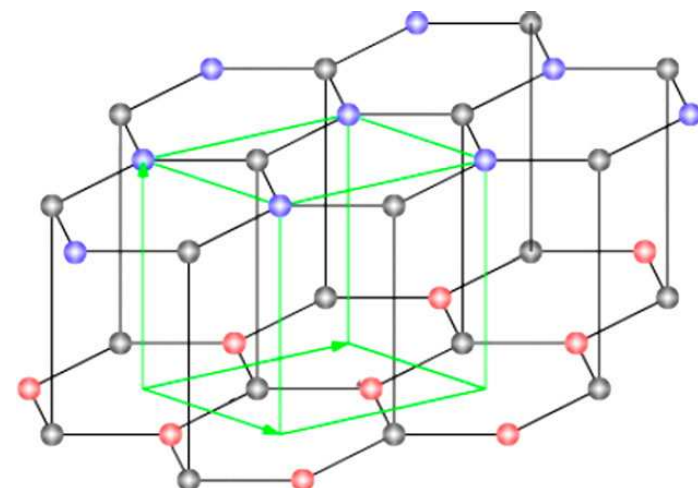
Rys. 2. Model struktury grafenu (Vozmediano 2011)
