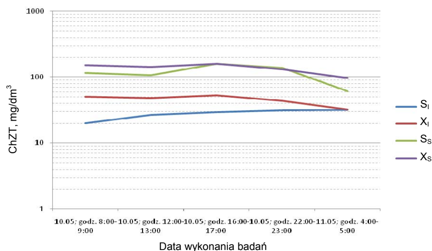
Rys. 3. Zmiany stężenia frakcji ChZT ( S_i , X_i , S_s , X_s ) w ściekach po oczyszczaniu mechanicznym – próbki chwilowe, godzinowe (skala osi rzędnych jest skalą logarytmiczną)
