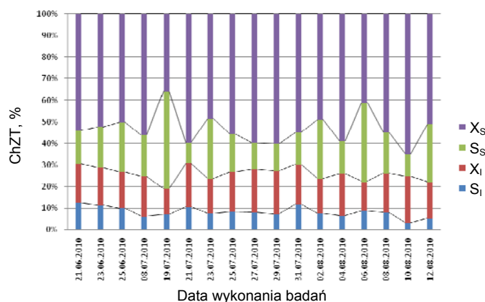
Rys. 10. Procentowy udział frakcji ChZT ( S_i , X_i , S_s , X_s ) w ściekach dopływających – wartości średniodobowe
