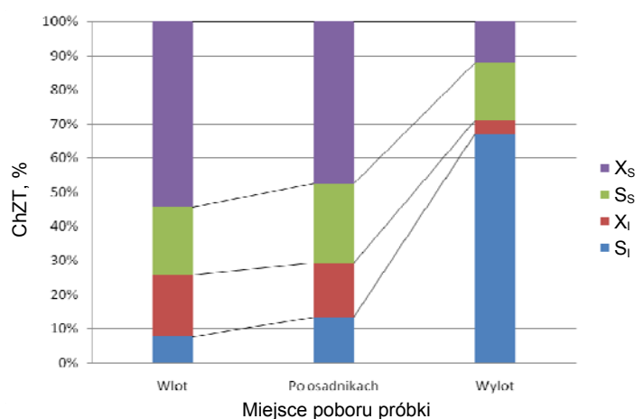
Rys. 17. Procentowy udział frakcji ChZT ( S_l , X_l , S_s , X_s ) po kolejnych stopniach oczyszczania – średnia dla wartości średniodobowych
