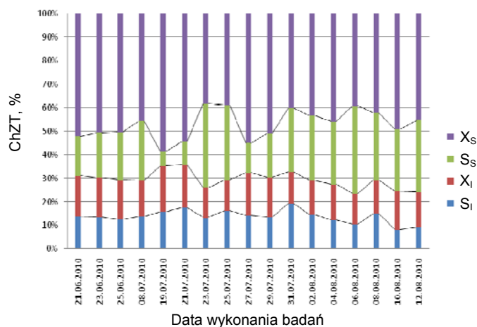
Rys. 12. Procentowy udział frakcji ChZT ( S_i , X_i , S_s , X_s ) w ściekach po oczyszczaniu mechanicznym – wartości średniodobowe
