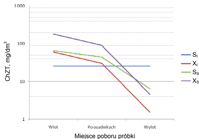
Rys. 16. Zmiany stężenia frakcji ChZT ( S_l , X_l , S_s , X_s ) po kolejnych stopniach oczyszczania – średnia dla wartości średniodobowych (skala osi rzędnych jest logarytmiczna)
