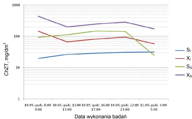
Rys. 1. Zmiany stężenia frakcji ChZT ( S_l , X_l , S_s , X_s ) w ściekach dopływających – próbki chwilowe, godzinowe (skala osi rzędnych jest logarytmiczna)
