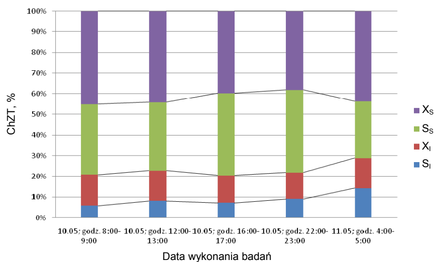
Rys. 4. Procentowy udział frakcji ChZT ( S_i , X_i , S_s , X_s ) w ściekach po oczyszczaniu mechanicznym – wartości średniodobowe – próbki chwilowe, godzinowe
