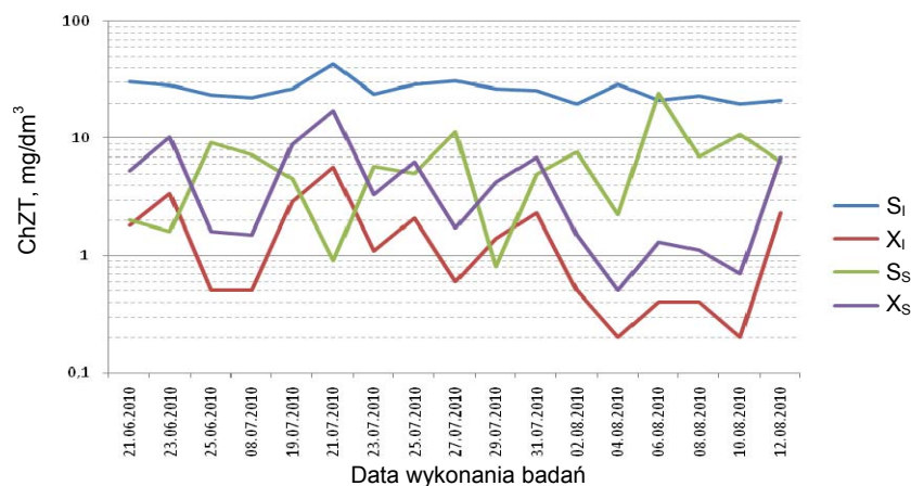
Rys. 13. Zmiany stężenia frakcji ChZT ( S_i , X_i , S_s , X_s ) w ściekach oczyszczonych (wylot) – wartości średniodobowe (skala osi rzędnych jest logarytmiczna)
