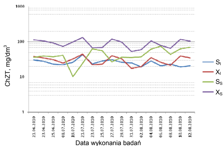
Rys. 11. Zmiany stężenia frakcji ChZT ( S_i , X_i , S_s , X_s ) w ściekach po oczyszczaniu mechanicznym – wartości średniodobowe (skala osi rzędnych jest skalą logarytmiczną)
