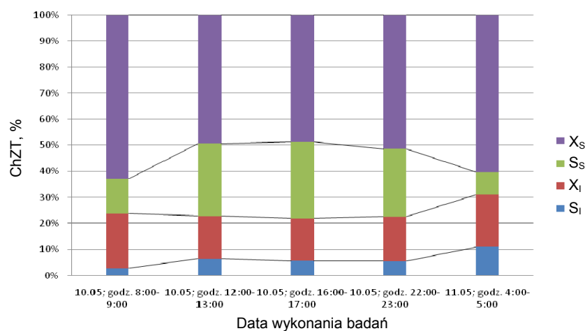
Rys. 2. Procentowy udział frakcji ChZT ( S_l , X_l , S_s , X_s ) w ściekach dopływających – próbki chwilowe, godzinowe
