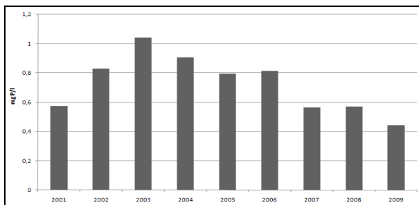
Stężenie fosforu ogólnego w Bierawce 32 km w latach 2001–2009
