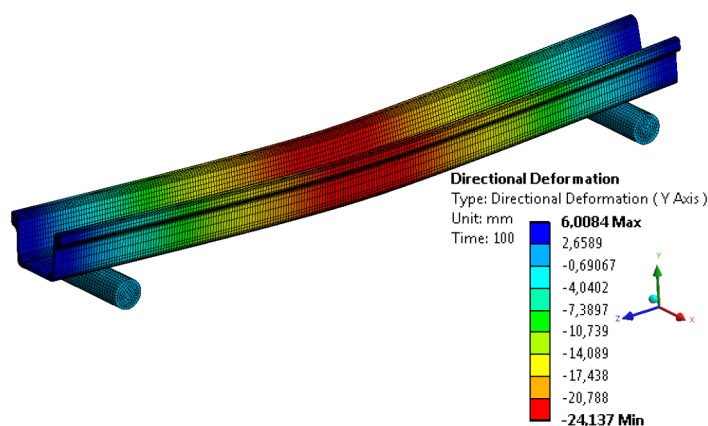
Rys. 12. Deformacje prostego odcinka kształownika KO „dnem w dół”; przemieszczenia [mm], skala \times 1
