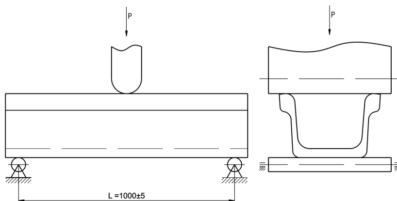
Rys. 3. Schemat próby zginania „dnem w dół” prostych odcinków kształtowników
