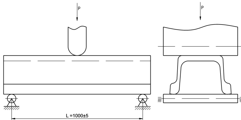
Rys. 4. Schemat próby zginania „dnem w górę” prostych odcinków kształtowników
