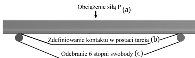
Rys. 10. Warunki brzegowe i sposób obciążenia modelu
