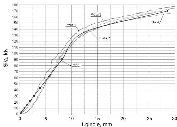
Rys. 13. Porównanie wyników stanowiskowych z wynikami uzyskanymi metodą elementów skończonych, wariant „dnem w górę”
