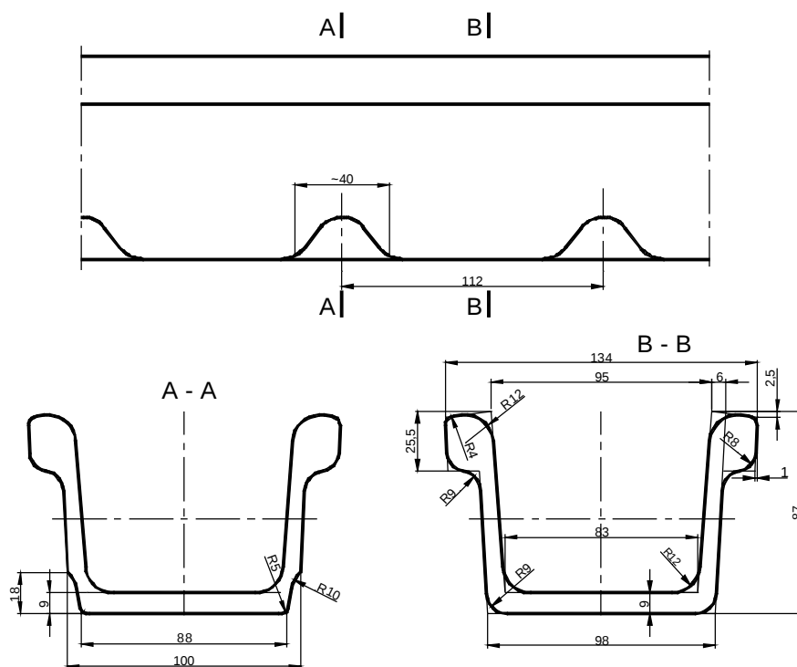
Rys. 2. Kształtownik KO21 na uniwersalne stropnice górnicze (USG)
