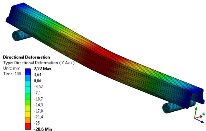
Rys. 11. Deformacje prostego odcinka kształownika KO21 „dnem w górę”; przemieszczenia [mm], skala \times 1
